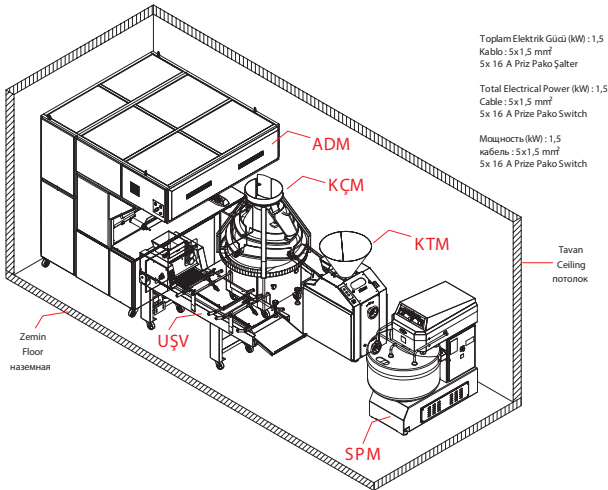
Perspektif Görünüş - Perspective View - Перспективный взгляд
