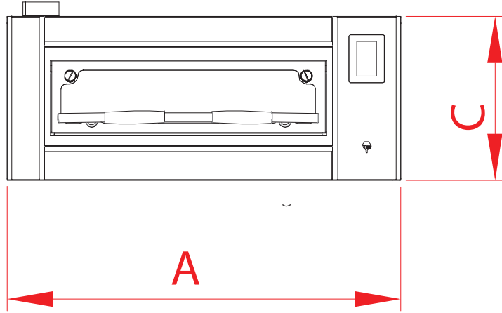
Sol Yan Görünüş - Left Side View - слева Вид сбоку
