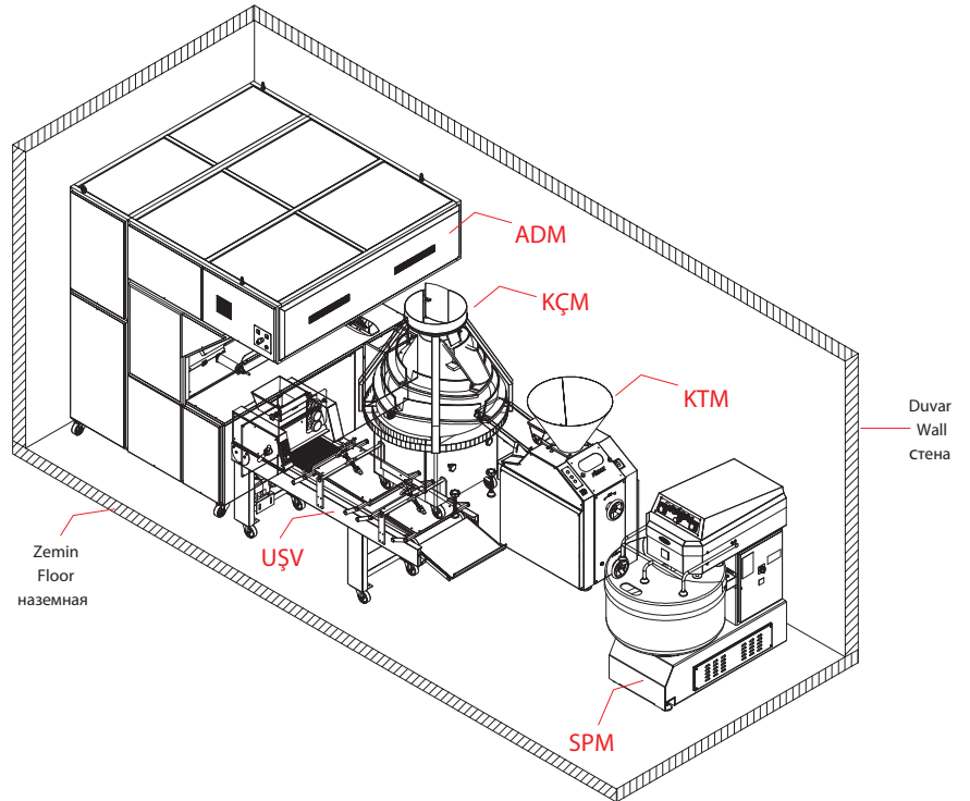
Perspektif Görünüş - Perspective View - Перспективный взгляд
