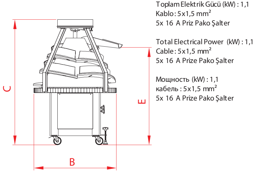
Sol Yan Görünüş - Left Side View - слева Вид сбоку
