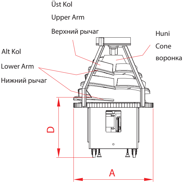
Ön Görünüş - Front View - вид спереди
